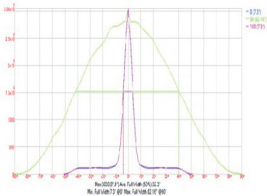
Işık Dağılım Grafiği (Yayılım Açısı 7.30 derece)
